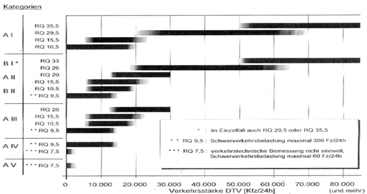
Abbildung 1: Einsatzbereiche von Querschnitten der RAS-Q (gültig bis 2008)
